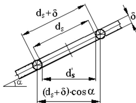
Fig. 4. Reducerea aparentă a deschiderii ochiurilor sitei ca urmare a înclinării acesteia.
