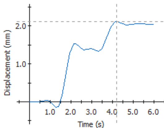
Fig. 2. Cursa de translație a bielei de-a lungul axei mașinii-reprezentare grafică
