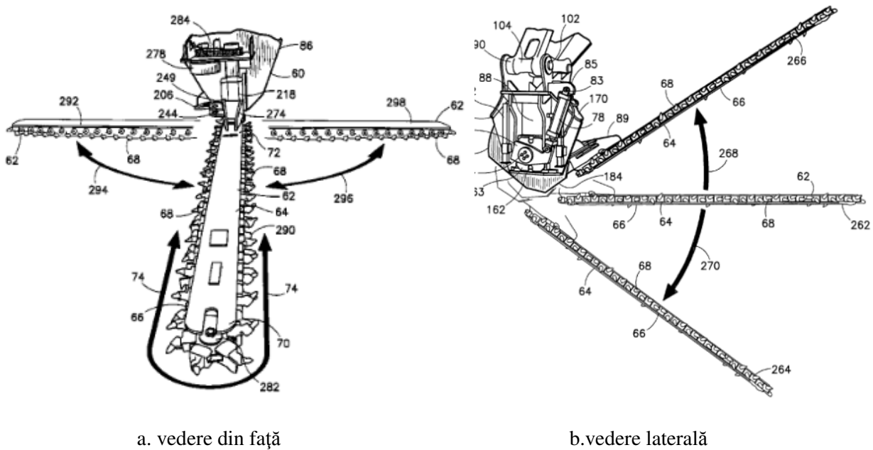
Fig. 3. Echipament pentru extragerea pietrei sparte prevăzută cu lanț port-dinți [7]
