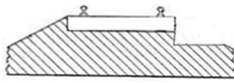
b. excavarea zonei de la capetele traverselor folosind utilaje uzuale (ex. excavatoare)
