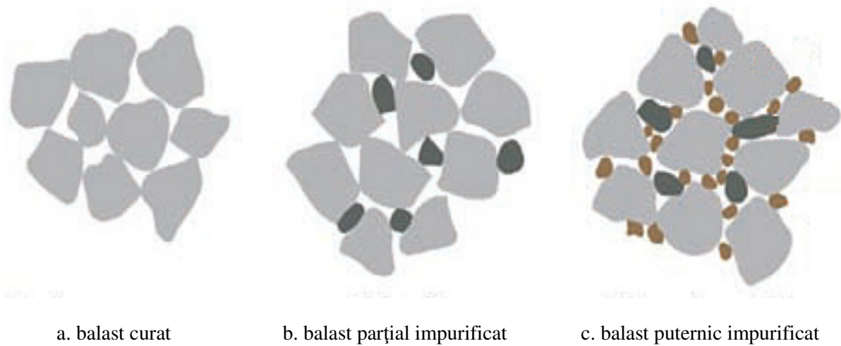
Fig. 1. Stadii specifice ale materialului prisme de balastare în timpul exploatării căii
