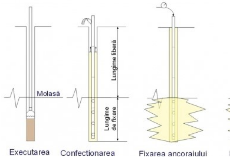
Figura 1. Etapele tehnologice parcurse pentru realizarea lucrărilor de consolidare cu micropiloți
